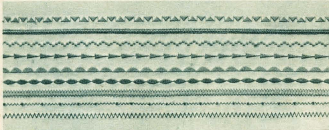
Siersteken, die door rhythmisch bewegen van de zigzag-knop ontstaan.
