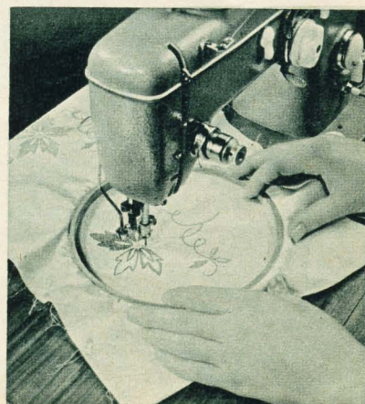
Hier ziet U de werkwijze van de knoopjessteek.
